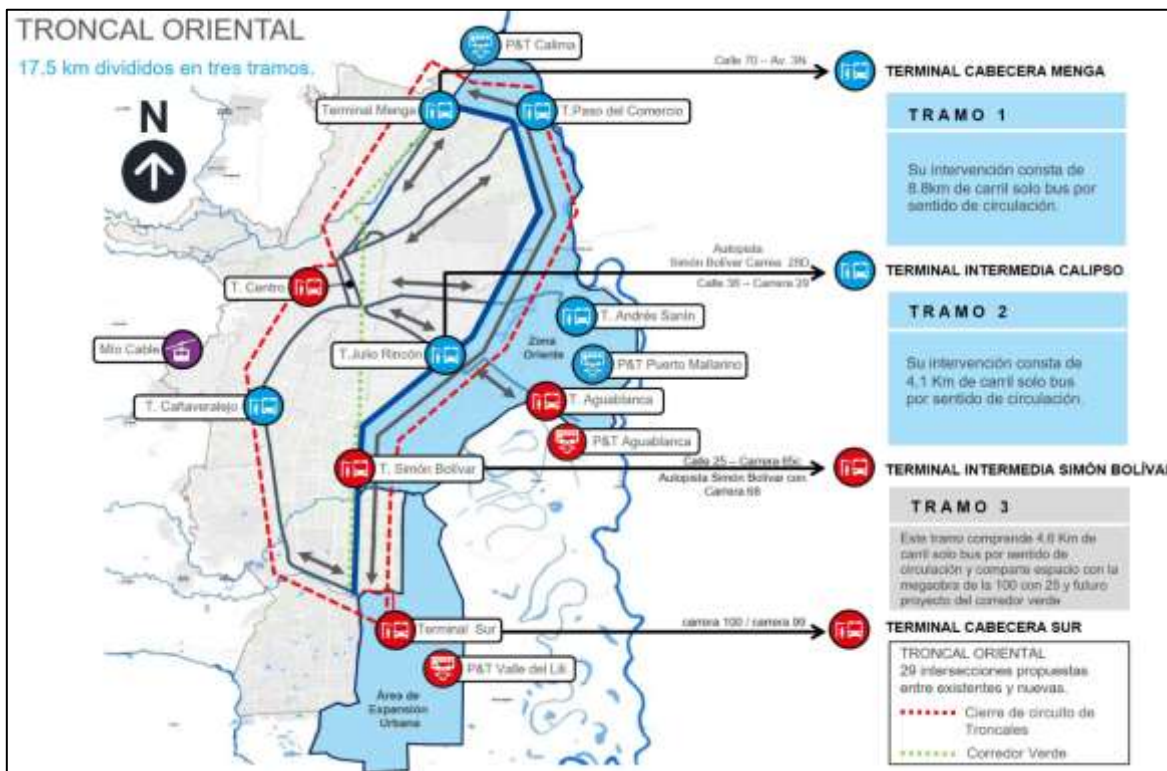
Figura 4. Localización y delimitación de los 3 tramos de la Troncal Oriental
