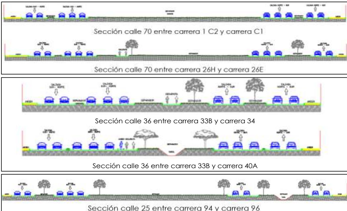
Figura 5. Secciones típicas de los tramos
