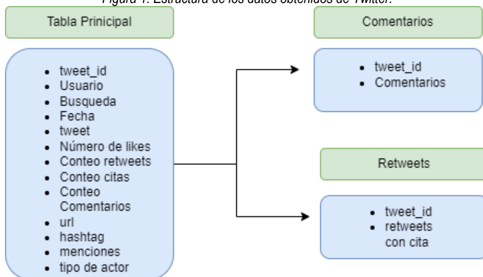
Figura 1: Estructura de los datos obtenidos de Twitter.
